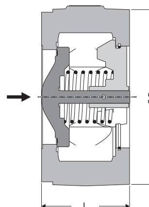
DN 80-200
