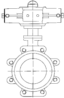
MR manual actuator
