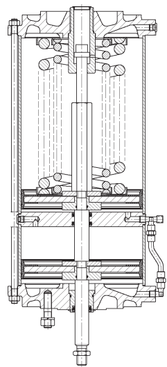
type LAP-SF (double piston)
